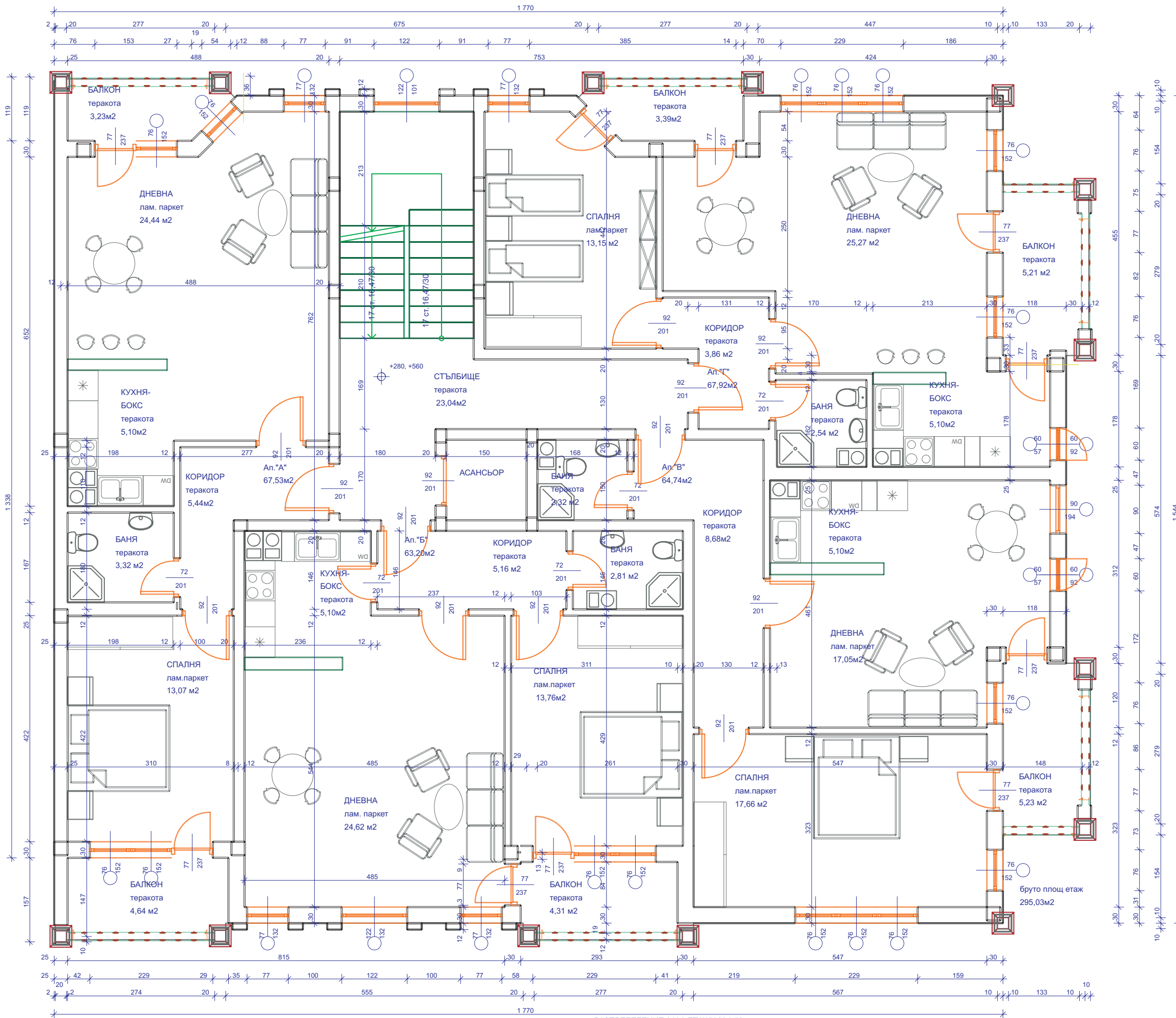
РАЗПРЕДЕЛЕНИЕ 2 И 3 ЕТАЖИ М 1:50
