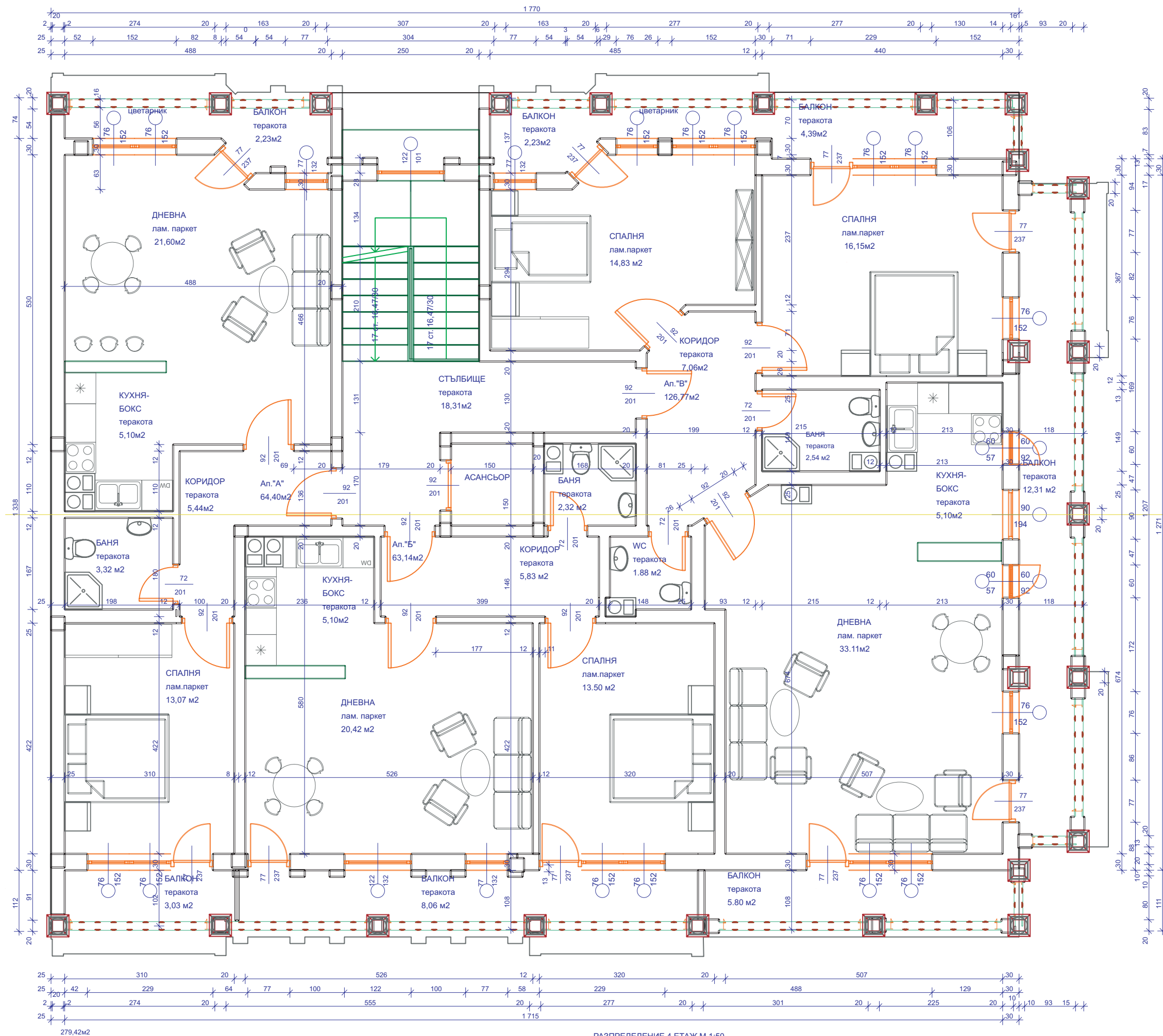
РАЗПРЕДЕЛЕНИЕ 4 ЕТАЖ М 1:50
